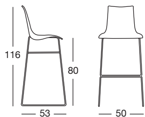
Struttura a slitta Sledge frame Art. 2542
