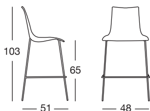
h.65 struttura a 4 gambe h.65 4-leg frame Art. 2541
