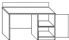
Стол рабочий ГСР 1200x600x(750+120)
