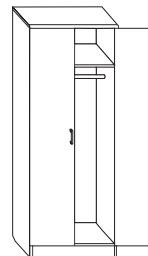
Шкаф комбинированный ГШК 900x600x2100
