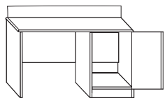
Стол с тумбой под холодильник ГСП(Л) 1200x600x(750+120)
